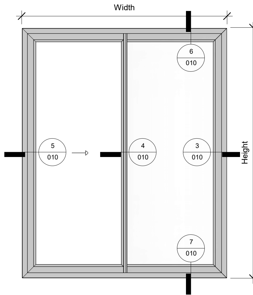
2 Elevation Back 1 : 20
