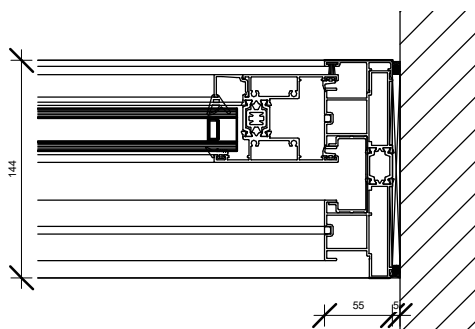
5 Detail 3 1 : 5
