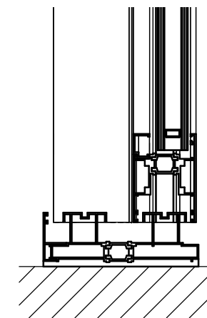
7 Detail 5 1 : 5
