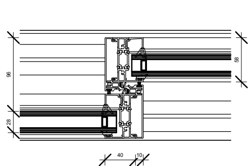
4 Detail 2 1 : 5
