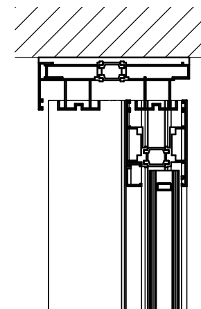
6 Detail 4 1 : 5
