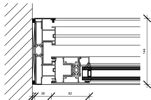
3 Detail 1 1 : 5
